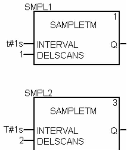
Рис.2.18. Використання 2-х екземплярів SAMPLETM зі зсувом на один цикл відносно один одного
