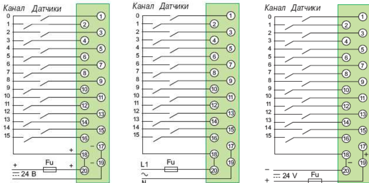
Рис.1.9. Підключення модулів дискретних входів зі з'ємними колодками.
